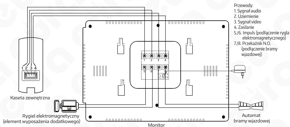
Rys. 6. Schemat połączeń zestawu
