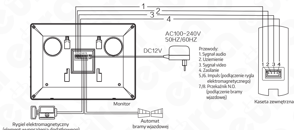
Rys. 6. Schemat połączeń zestawu
