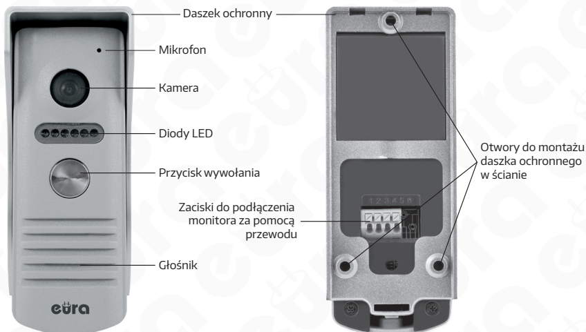
Rys. 2 Budowa kasety zewnętrznej VDA-10A3
