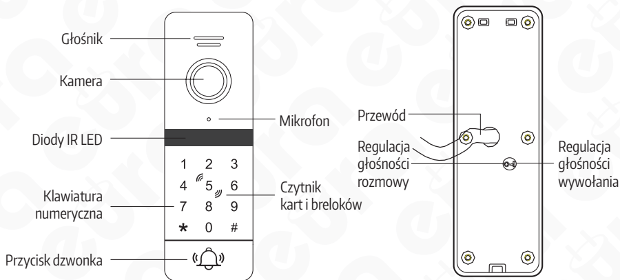
Rys. 1 Budowa kasety zewnętrznej
