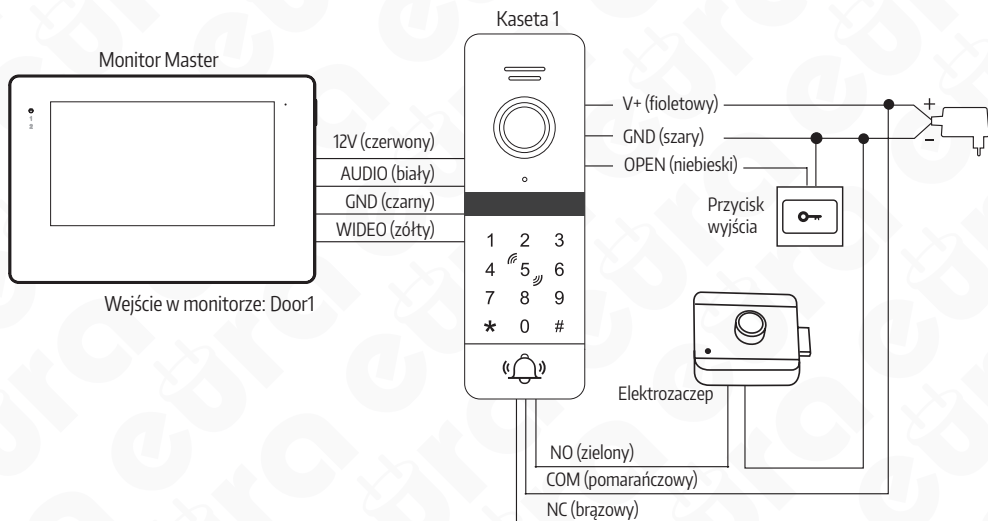
Rys. 4. Schemat połączeń dla elektrozaczepek zwykłego
