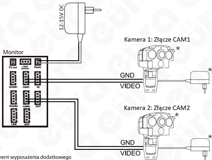
Rys. 7. Schemat połączenia dodatkowych kamer
