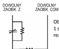
Rysunek 1-4 Podwójne rezystory końcowe
