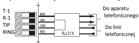
Rysunek 1-6 Podłączenie linii telefonicznej
