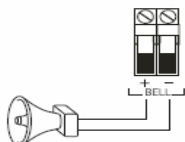
Rysunek 1-5 Podłączenie urządzeń do wyjścia BELL
