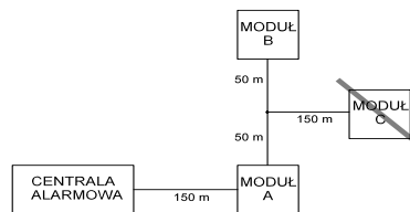
Rysunek 1-1 przykład podłączenia modułów i klawiatur do magistrali Corbus przedstawia umieszczony rysunek. Urządzenie (A) zostało podłączone prawidłowo, ponieważ jego odległość od magistrali nie przekracza 305m, podobnie urządzenie (B), urządzenie (C) zostało podłączone niepoprawnie ponieważ jego odległość od magistrali przekracza dystans 305m.
